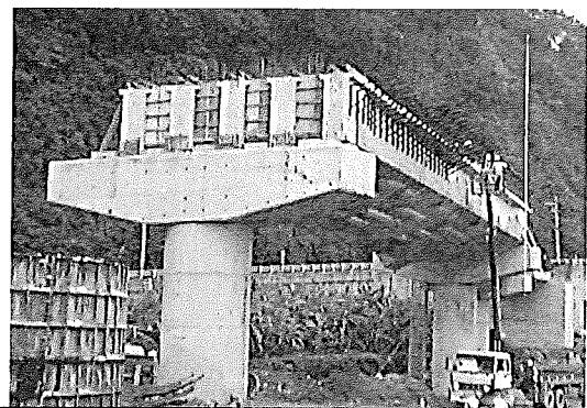
照片 10：預力梁吊放後隔梁施工中
