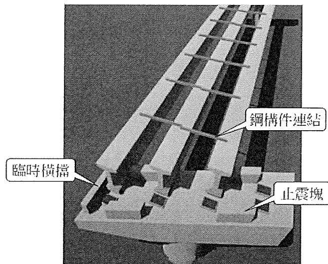
圖 7 止震塊示意圖
