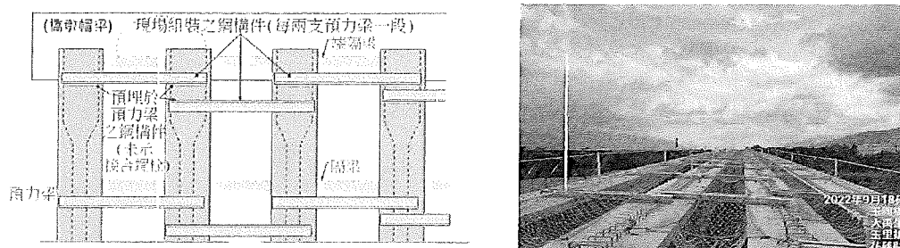
圖 5 鋼構件連接平面配置方式及實際案例
