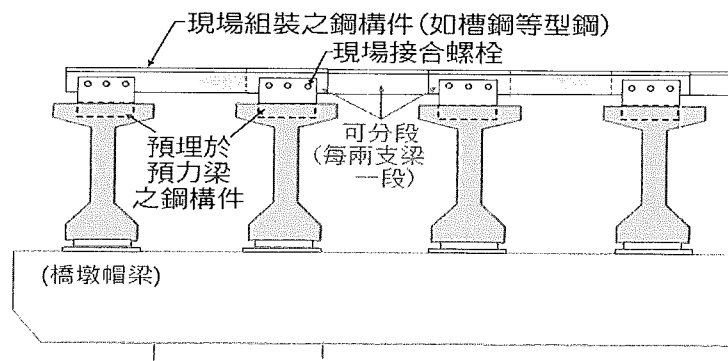
圖 10 鋼構件連結設置示意圖
