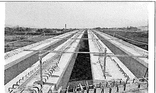
照片 8：吊放後-木料角材橫向連結
