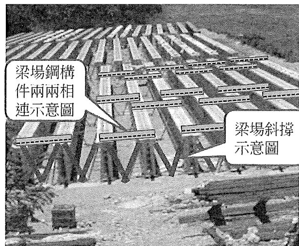
圖 9 梁場妥善固定預鑄預力 I 型梁
