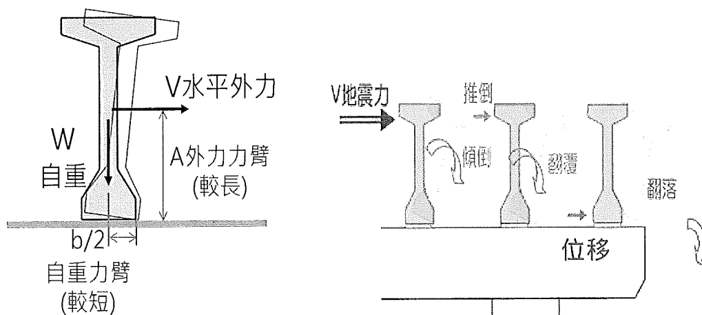
圖 1 預力 I 型梁易產生翻覆傾倒或位移掉落
