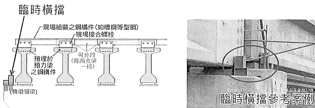
圖 6 帽梁外側設置臨時橫擋
