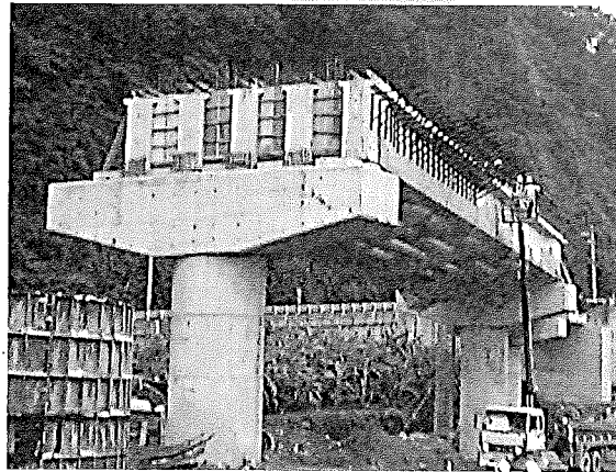
圖 11 端隔梁現場施工圖
